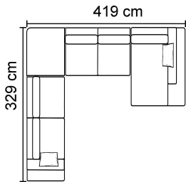
135 SECT.(16+229+28+49)
